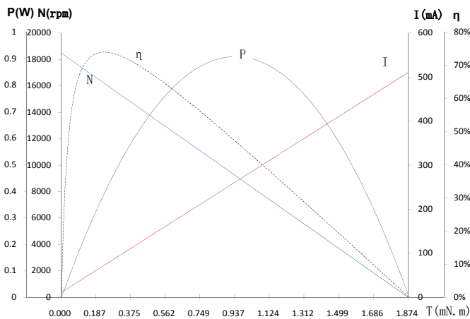
型号 / Model L1213N5M01-185-7.4
