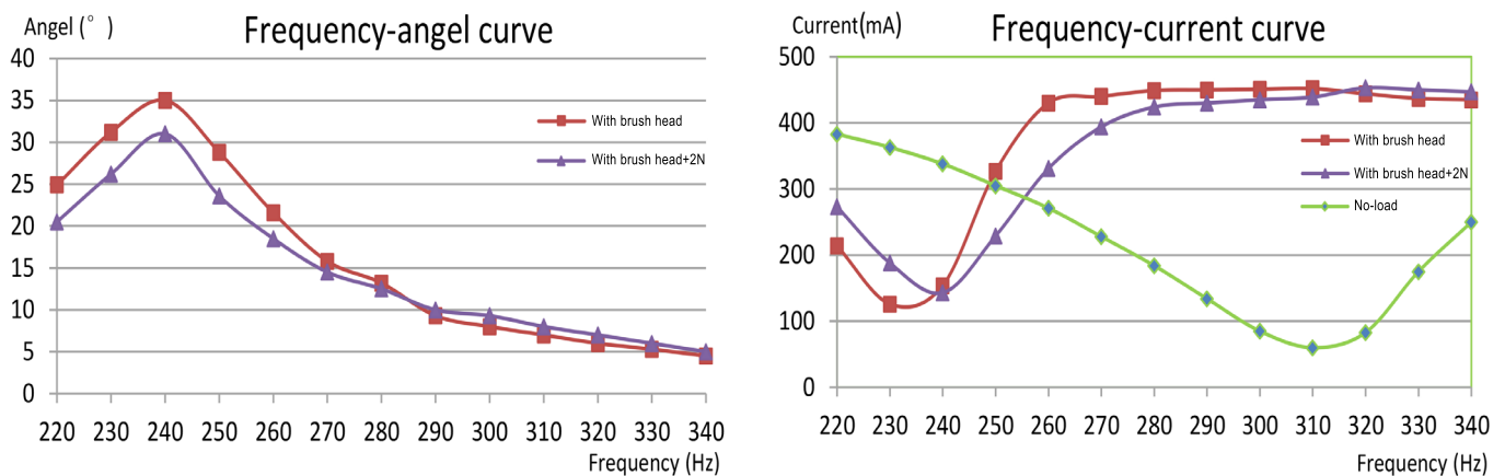
型号 / Model 1941ZDF-1-L3-3.7
