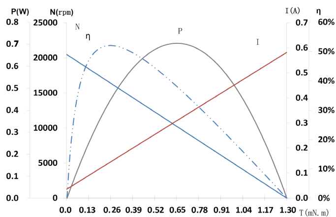
型号 / Model C1015F33-0107
